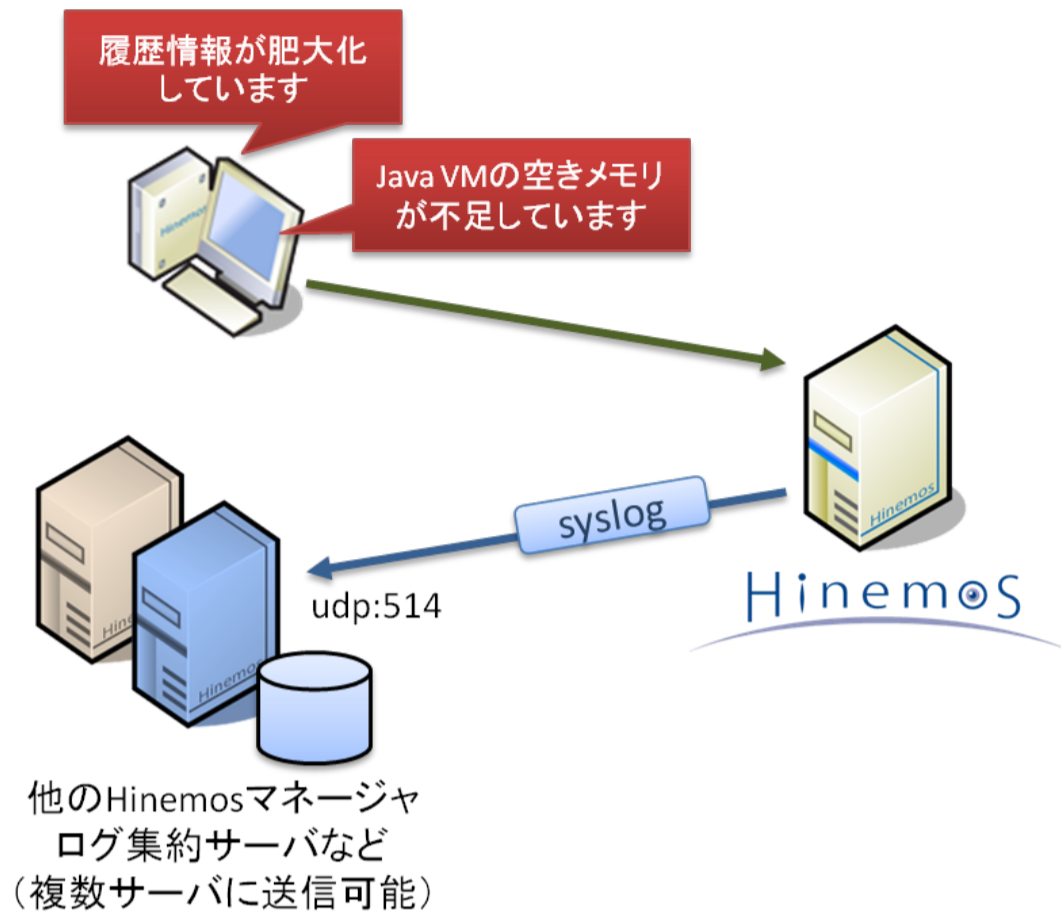
図5-3. セルフチェック機能の概要
