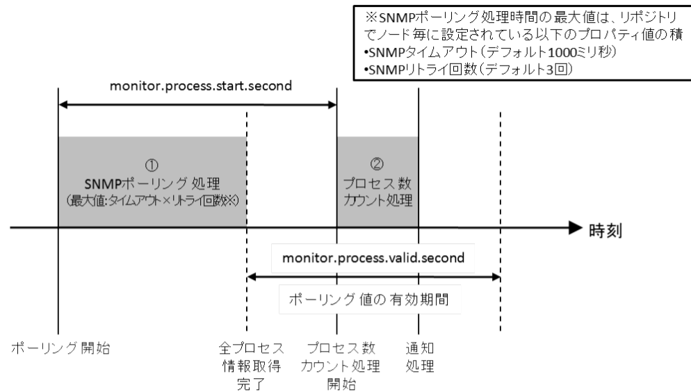
図 7-1 プロセス監視の処理
