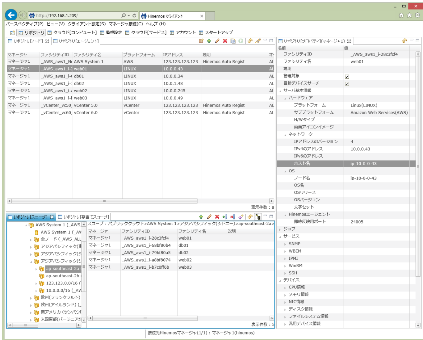
図4-3 リポジトリパースペクティブ
