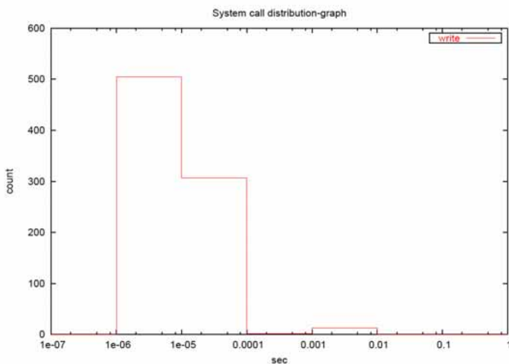
図 14 write システムコール時間分布の可視化例
