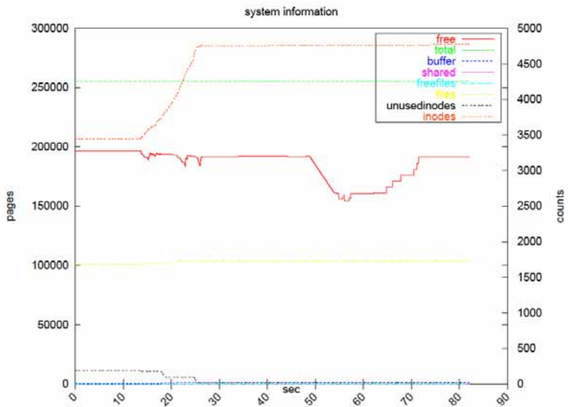
図 16 カーネル状態変化の可視化例
