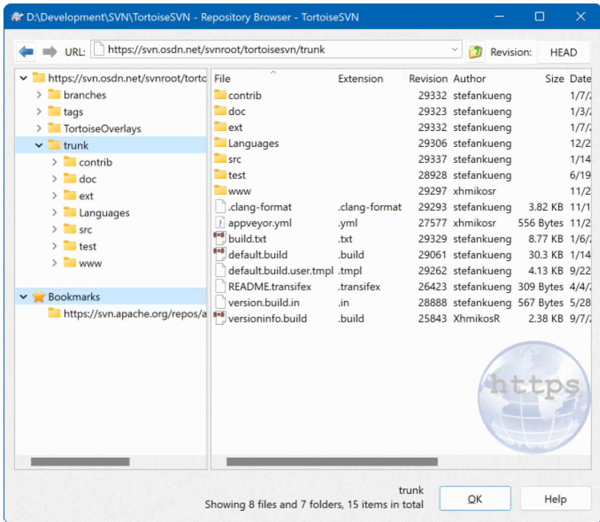
Obrázok 4.62. Prehliadač úložiska
