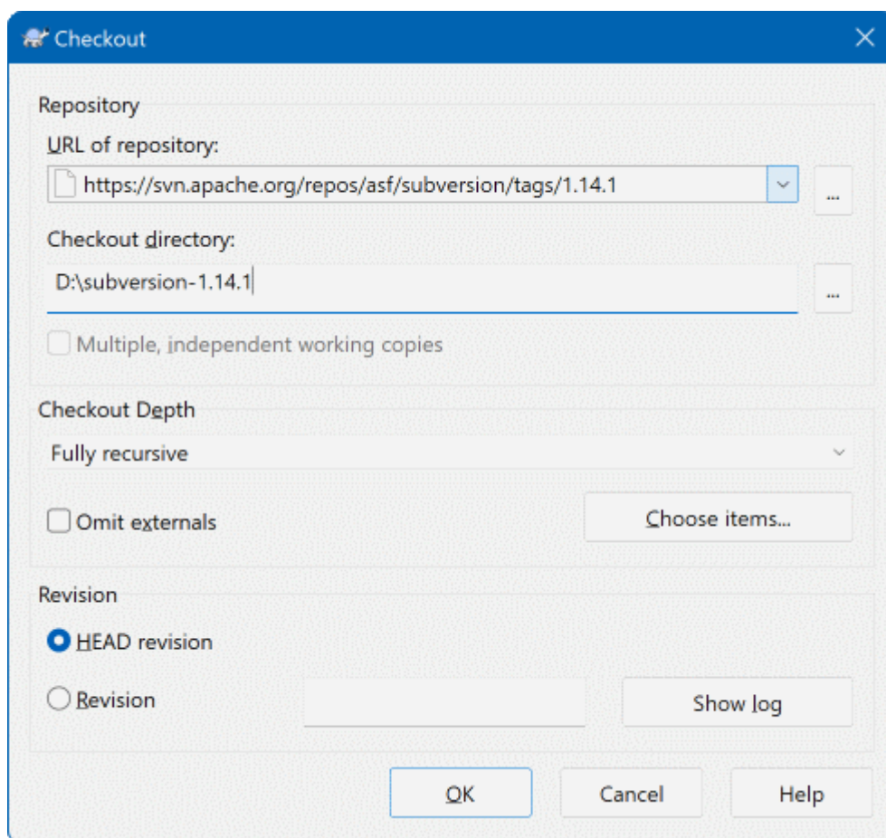
Obrázok 4.7. Dialóg overenia
