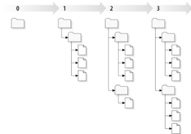
Obrázok 2.7. Úložisko
