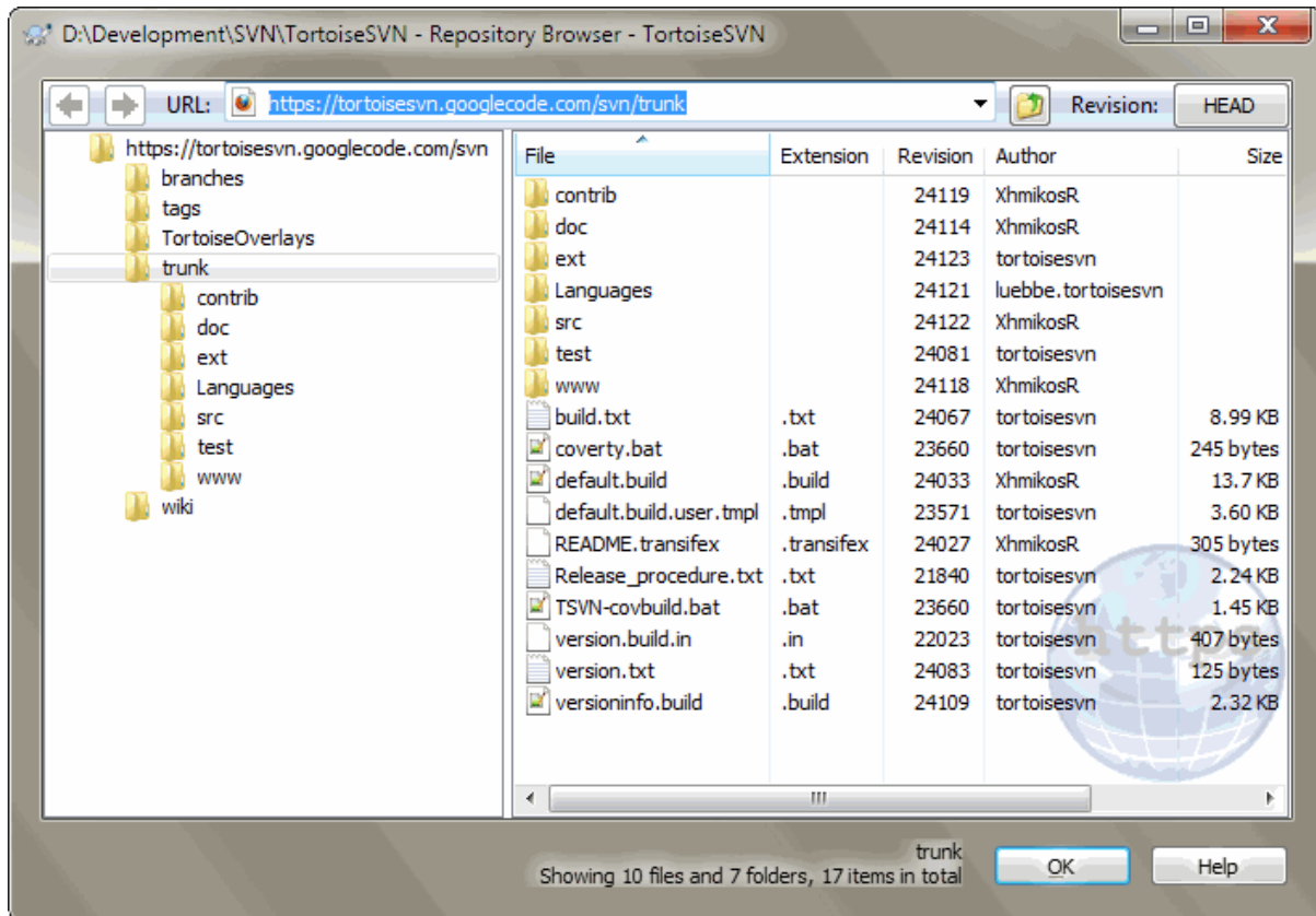
Gambar 4.62. Browser Repositori
